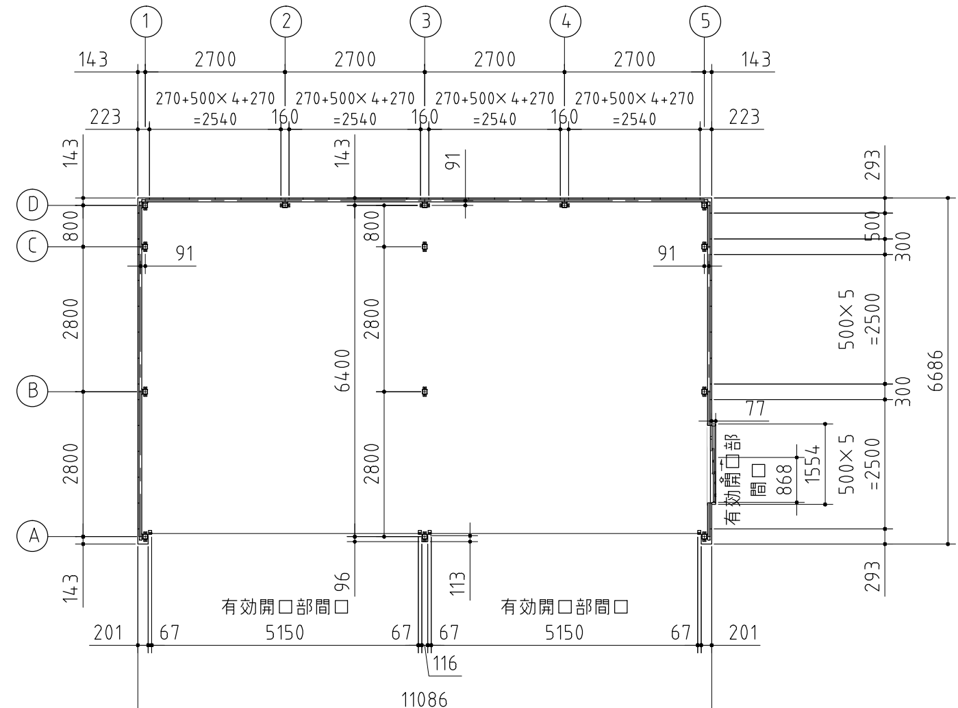
平面図
